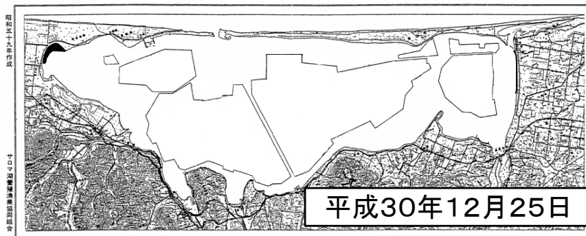
サロマ湖結氷状況
