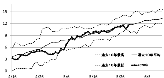
2020年サロマ湖水温(中央部)
