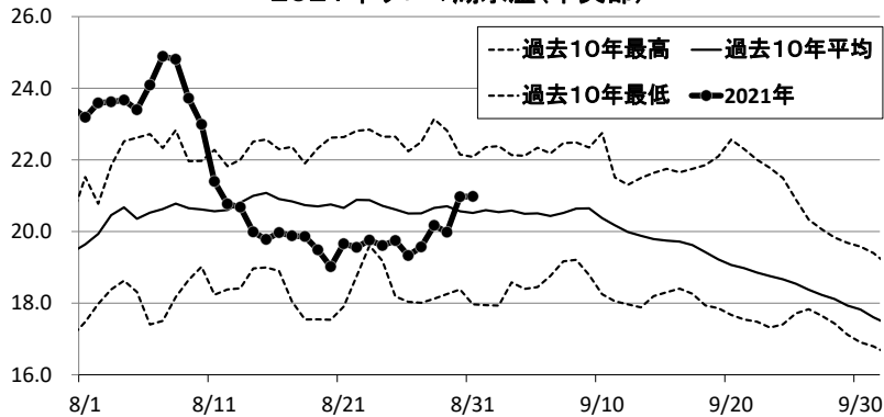
2021年サロマ湖水温(中央部)
