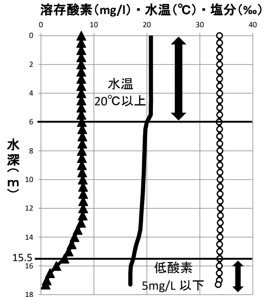
2021年サロマ湖水温(中央部)
